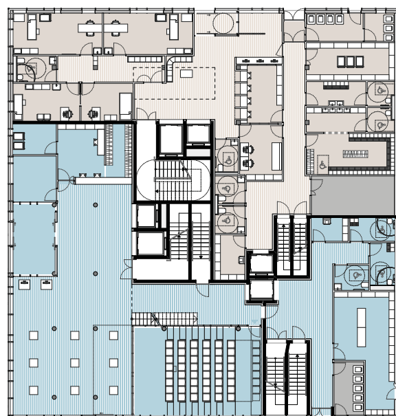
RDC
